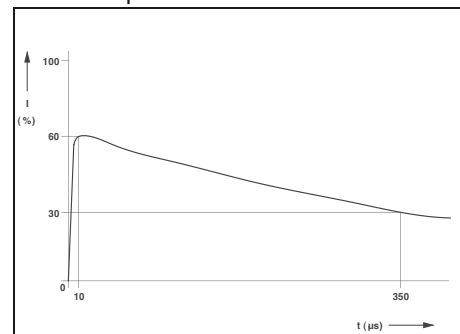
Импульс тона молнии формы 10/350 согласно МЭК 62305-1
