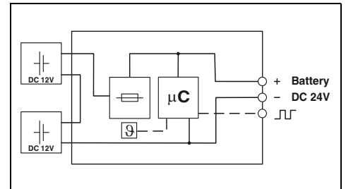
Энергоаккумулятор с расширенным температурным диапазоном, 24 В пост. тона, 26 Ач
