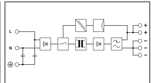
Источник питания, однофазный, 12 В пост. тока, 5 А
