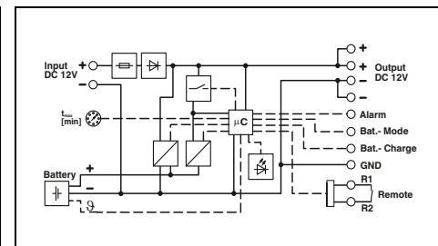
Источник бесперебойного питания со встроенным аккумулятором 12 В пост. тона / 12 В пост. тона, 4 А
