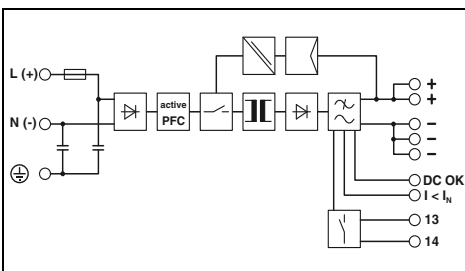
Источник питания, однофазный, 24 В пост. тока, 20 А
