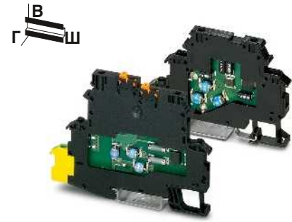
Витая пара (петля), без потенциала земли
