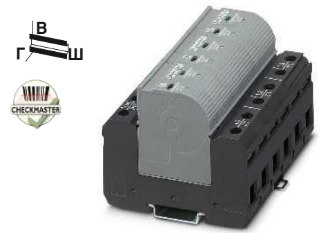
4-проводная система, L1, L2, L3, PEN
