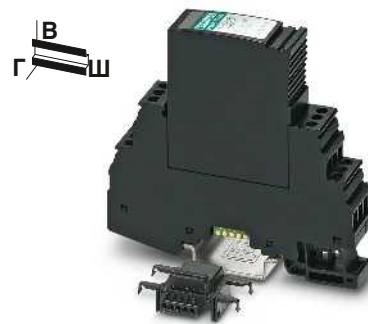
2 проводника, с общим опорным потенциалом, соединение 9/10 заземлено через газовый разрядник
