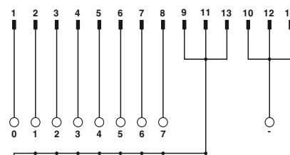
Схема подключения VIP-2/.../FLK14/8P/PLC
