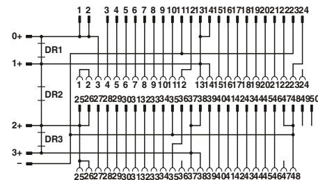
Схема подключения FLKM 50-PA-S400
