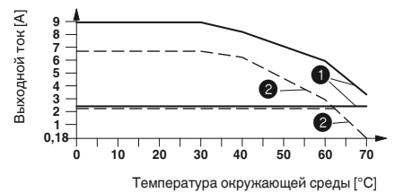
Кривая измерения характеристик ELR H5-I-SC-24DC/500AC-2 и ELR H5-I-SC-24DC/500AC-9 Продолжительность включения 100 %
