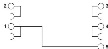
Схема подключения PLC-VT/АКТ
