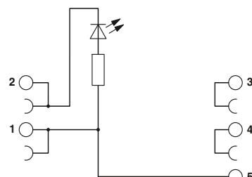
Схема подключения PLC-VT/АКТ/LA
