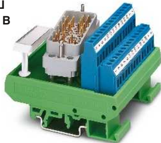
25-контактная
