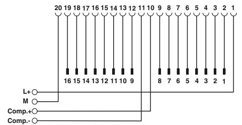
Схема подключения FLKM 16-PA-S300/MINI-MCR
