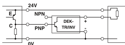
Выход p-n-p-типа Нагрузка
