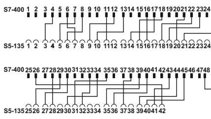
Схема подключения FLKM S135-470-4UC//S400
