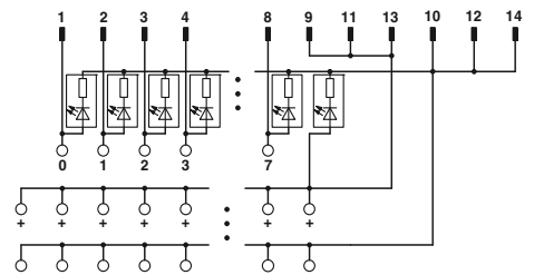
Схема подключения VIP-3/.../FLK14/8IM/LED/PLC
