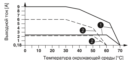
Кривая измерения характеристик ELR H5-I-SC-230AC/500AC-2 и ELR H5-I-SC-230AC/500AC-9 Продолжительность включения 100 %
