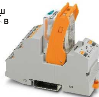
Релейный модуль RIF-2 с реле с 2 переключающими контактами
