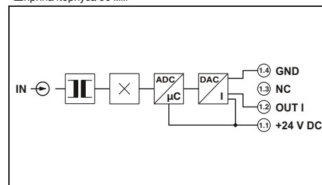
для постоянных, переменных и несинусоидальных токов от 0 до 600 А, Выход тока
