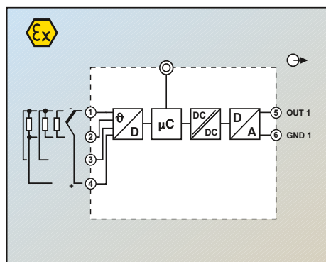
Блок-схема MCR-FL-T-LP-I-EX
