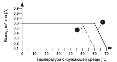
Кривая изменения характеристик ELR H5-I-SC-230AC/500AC-0,6 Продолжительность включения 100 %
