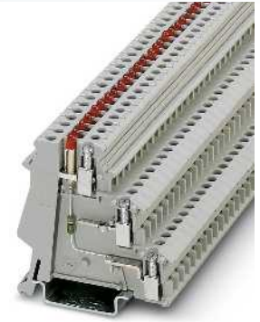
2,5 (4) мм 2 , 26 А, трехпроводная клемма со световым индикатором
