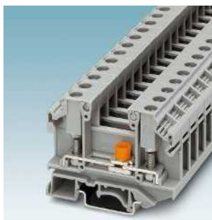
Болтовые клеммы с размыкателем OTTA 6-T
