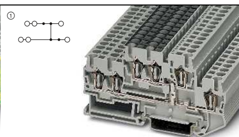
26 А, проходная клемма, с объединением потенциалов
