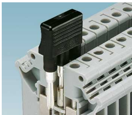
Короткозамыкающий штекер KSS ...
