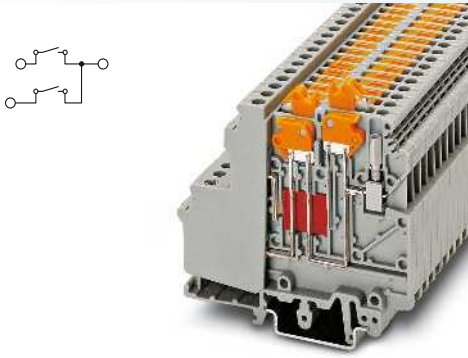
4 (4) мм 2 , 8 А, проходная клемма, 3 контакта, с двумя ножевыми размыкателями, винт с тестовым гнездом
