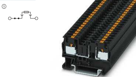
15 А, клеммы для плоских предохранителей типа F
