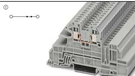
4 (4) мм 2 , 30 А, клемма, 1 проходной ярус L
