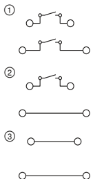
16 А, двухъярусная клемма с двумя разделительными зонами
