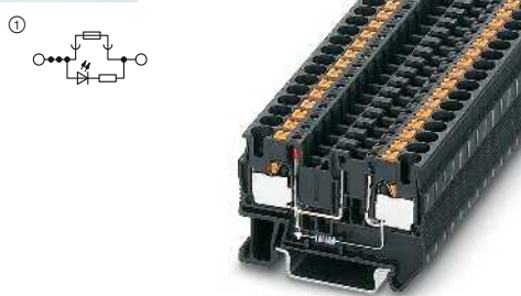
15 А, клеммы для плоских предохранителей типа F, с индикацией
