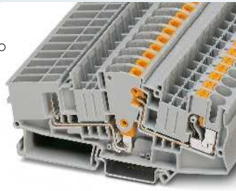
30 А, клемма для трансформатора тока, для короткозамыкающего штекера
