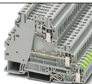
36 А, многоярусная клемма с разделительной зоной и основанием PE
