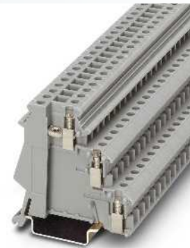
2,5 (4) мм 2 , 26 А, трехпроводная клемма для датчика
