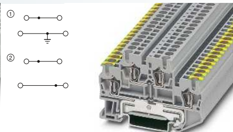
32 А, двухъярусная заземляющая клемма
