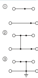
32 А, двухъярусные клеммы
