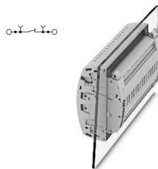
6 (10) мм 2 , 30 А, 4 ... 25-конт. базовый блок, для настенного монтажа, зажим push-in
