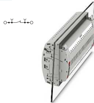
6 (10) мм 2 , 30 А, базовый блок, кодировка VDE тип B19
