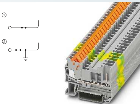
17,5 А, проходная клемма
