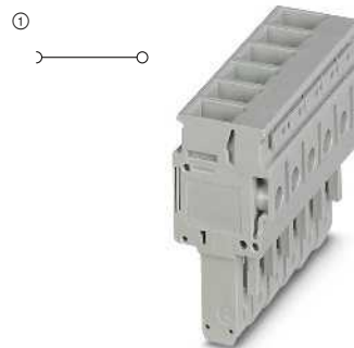
41 А, штекер, подключение в направлении проводника
