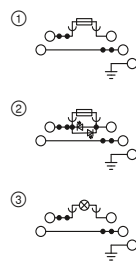
36 А, многоярусная клемма, с индикацией, под предохранитель, основание PE
