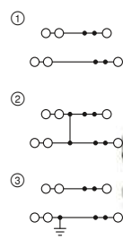
24 А, двухъярусная клемма, 3 контакта на ярус
