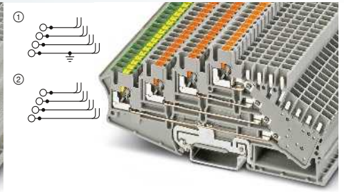
10 А, четырехъярусная клемма с заземляющим основанием
