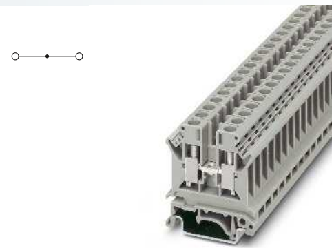
6 (10) мм 2 , 57 A, проходная клемма
