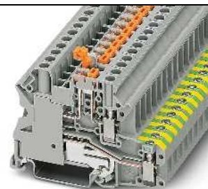
20 А, клемма с ножевым размыкателем и заземляющим контактом
