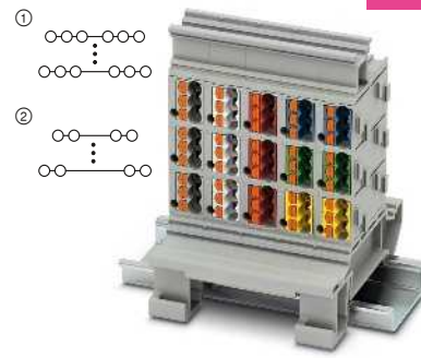
22 А, установка на монтажную рейку
