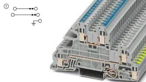
4 (4) мм 2 , 30 А, трехъярусная клемма, 1 проходной ярус L, 1 ярус N, 1 PE
