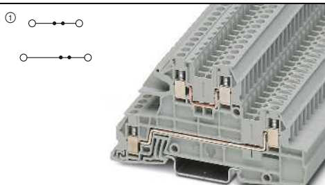
4 (4) мм 2 , 30 А, двухъярусная клемма, 2 проходных яруса L
