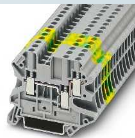
30 А, проходные и заземляющие клеммы, 3 контакта
