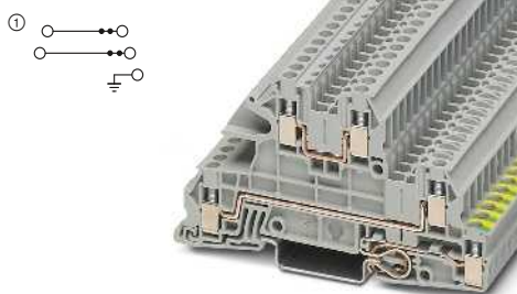
4 (4) мм 2 , 30 А, трехъярусная клемма, 2 проходных яруса L, 1 PE
