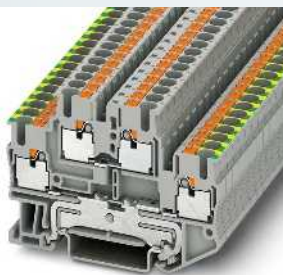
30 А, двухъярусная клемма с основанием PE
