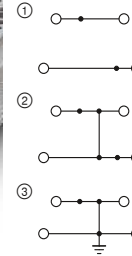
17,5 А, двухъярусные клеммы
