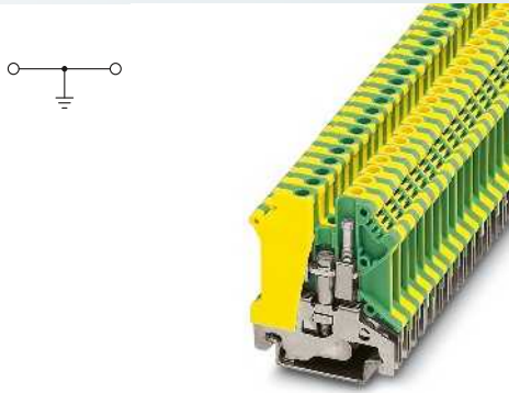
4 (6) мм 2 , заземляющая клемма
