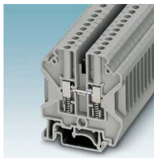
Винтовые клеммы с пружинной опорой USST ...
