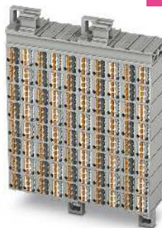
22 А, 80-элементов, 480 контактов, по 6 контактов на элемент
