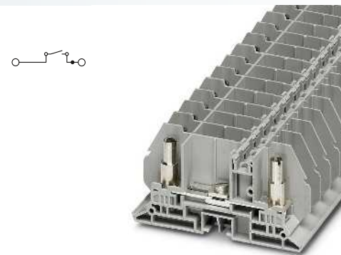
10 (10) мм 2 , 50 А, клемма с размыкателем для измерительного трансформатора, для непосредственного монтажа
