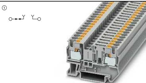
20 А, клемма с разрывом цепи
