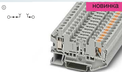
20 А, разделительная клемма, 3 функциональных отверстия и два контрольных гнезда 4 мм
