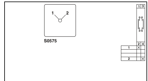
2,5 (2,5) мм 2 , 20 А, переключатель без положения 0, с гальванической развязкой контактов
