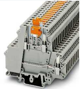
4 (4) мм 2 , 12 А, двухъярусная клемма с ножевым размыкателем винты с тестовым гнездом
