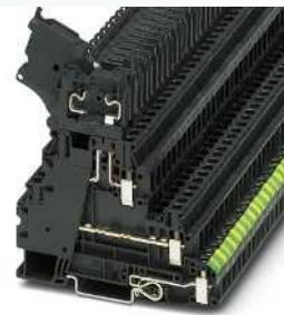
36 А, многоярусная клемма, с индикацией, под предохранитель, основание PE
