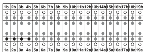
Тестовый штекер типа B19
