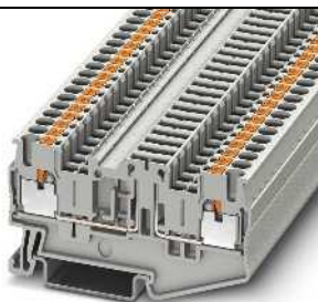
16 А, клемма с разрывом цепи, 4 функциональными отверстиями
