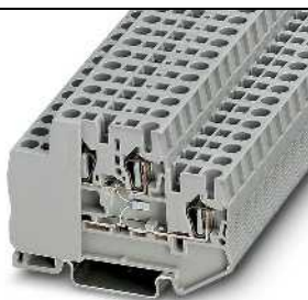
26 А, двухъярусная клемма с датчиком температуры
