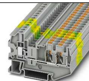
38 А, проходная клемма, 3 контакта
