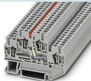
26 А, двухъярусная клемма со световым индикатором
