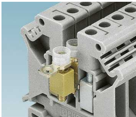
Винтовая перемычка с изоляцией ISSBI ...
