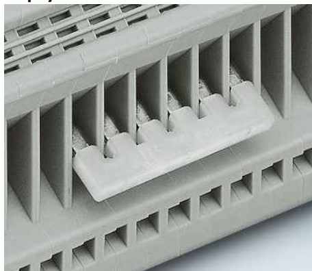
Перемычка для цепи "треугольник" EB .../DR
