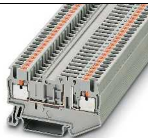
20 А, клемма с разрывом цепи, 2 функциональными отверстиями
