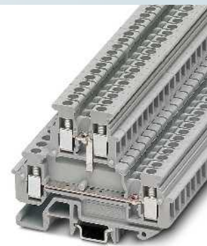
2,5 (4) мм 2 , 24 А, двухъярусная клемма для впаики компонентов
