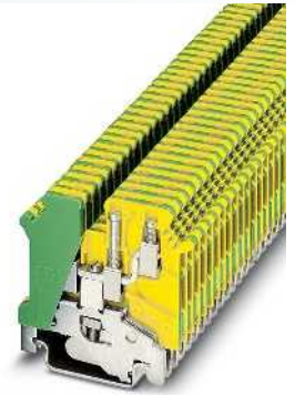
2,5 (2,5) мм 2 , заземляющая клемма, 3 контакта
