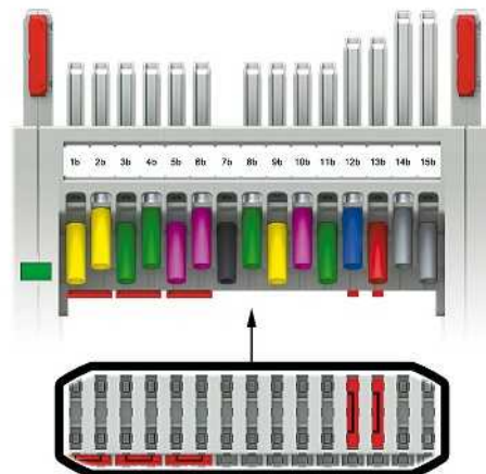
Тестовый штекер с трансформатором тока, напряжения и сигналов
