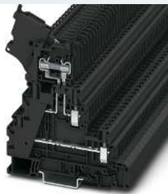
36 А, многоярусная клемма, под предохранитель
