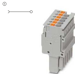
17,5 А, штекер, подключение в направлении проводника
