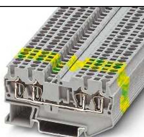
17,5 А, проходная клемма, 4 контакта
