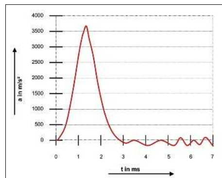
Диаграмма удара в течение 3 мс/350 g
