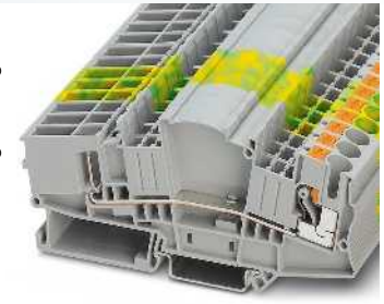
30 А, проходная клемма, для короткозамыкающего штекера
