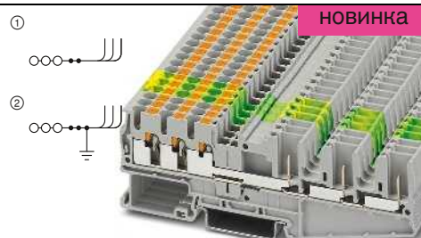
24 А, проходная клемма, 6 контактов
