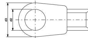
Кабельный наконечник DIN 46234: 1980-03
