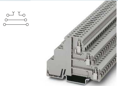
2,5 (4) мм 2 , 30 А, трехъярусная клемма с зоной разделения
