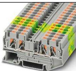
38 А, проходная клемма, 4 контакта
