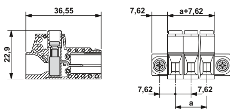
Тип: IPC 5/...-ST-7,62 с PC 5/...-ST1-7,62 Сечение провода: 6 мм 2
