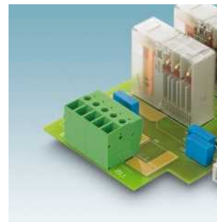
Серия FRONT 4: фронтальные винтовые разъемы, до 32 А, подключение: вертикальное, шаг 6,35 / 7,62 мм FRONT 4 V... Стр. 459
