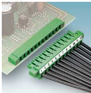
Штекеры с винтовыми зажимами и ответные части, шаг выводов 5,08 мм MC 1,5/...-ST(F)-5,08 Стр. 246
