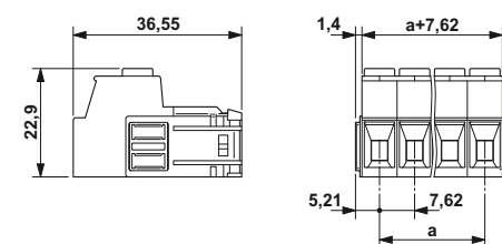
Тип: IPC 5/...-ST-7,62 с IPC 5/...-G-7,62 Сечение кабеля 6 мм 2
