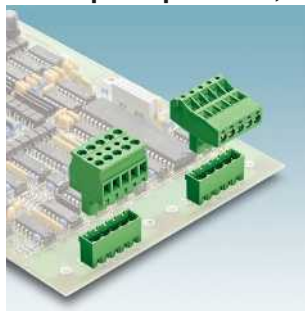
Штекеры TWIN с винтовыми зажимами, шаг выводов 5,08 мм, для разветвления цепей TMSTBP 2,5/...-ST(F)-5,08 Стр. 270
