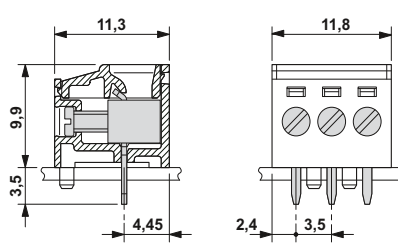
MKDSFW 1,5/3-3,5 (с опорным штифтом), см. стр. 87.
