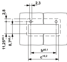
Размер выреза для DFK-MS 1,5/...-GF, см. стр. 240.
