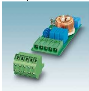
Серия PC 16: штекеры со двоянными винтовыми зажимами, до 76 А, шаг 10,16 мм TPC 16... Стр. 556
