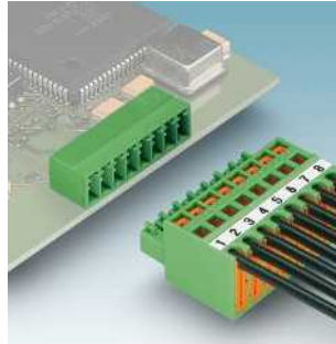
Штекеры с прокалывающими контактами, шаг 3,81 мм, сечение провода 0,5 мм 2 QC 0,5/...-ST(F)-3,81 Стр. 204
