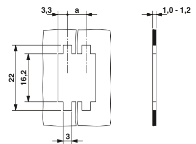
Проходная деталь CIOC...FL, см. стр. 65. Размер a = 6,5 мм
