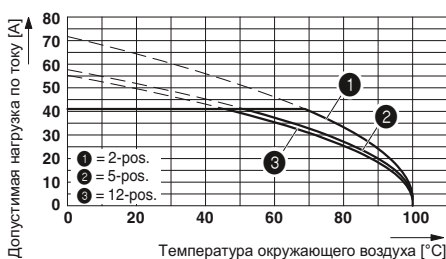
Тип: IPC 5/...-ST-7,62 с IPC 5/...-G-7,62 Сечение кабеля = 10 мм 2
