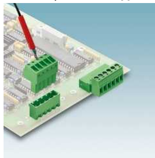
Штекеры с винтовыми зажимами, шаг выводов 5,0 / 5,08 мм, с стетовым гнездом или без него MSTB 2,5/...-ST(F)-... Стр. 262
