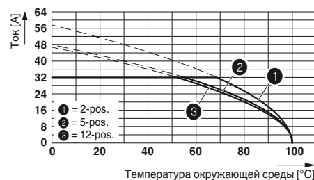
Тип: IPC 5/...-ST-7,62 с IPC 5/...-G-7,62 Сечение кабеля 6 мм 2
