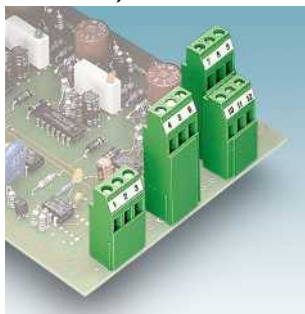
Высокие клеммы для печатных плат, с шагом 5,0 / 5,08 мм MKKDSNH 1,5/...-5,08 Стр. 93 MK3DS 1,5/...-5,08-BC Стр. 99
