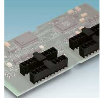
Ответные части, для пайки оплавлением припоя, шаг выводов 3,5 / 3,81 мм, подключение параллельно или перпендикулярно печатной плате Стр. 208
