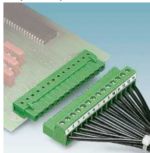
Инвертированные штекеры с винтовыми зажимами, шаг выводов 5,08 мм IC 2,5/...-ST(F)-5,08 Стр. 272
