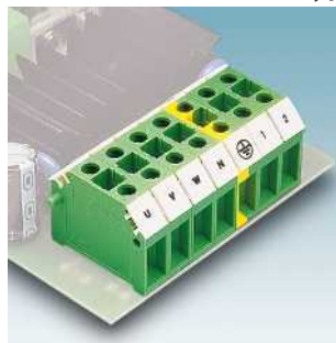
Серия KDS 10: проходные клеммы с винтовыми зажимами, до 76 А, шаг 10 мм KDS 10/... Стр. 457
