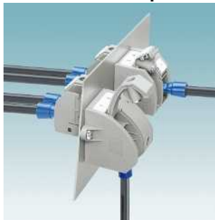
Серия RW 5: болтовые разъемы, до 76 А, подключение: вертикальное и горизонтальное RW 5... Стр. 624
