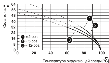
Тип: IPC 5/...-ST-7,62 с PC 5/...-ST1-7,62 Сечение провода: 6 мм 2
