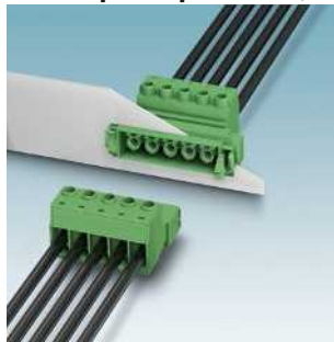
Серия PC 16: инвертированные проходные ответные части, с выводами под пайку и винтовыми зажимами, до 76 А, шаг 10,16 мм DFK-IPC 16... Стр. 578
