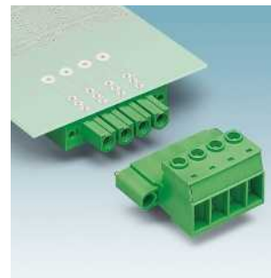
Серия PC 16: инвертированные штекерные/ответные части, винтовые зажимы, до 76 А, шаг 10,16 мм IPC 16/... Стр. 558
