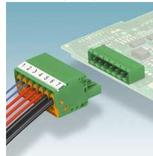
Штекеры с прокалывающими контактами, шаг 5,0 / 5,08 мм QC 1,0/...-ST(F)-5,08 Стр. 290 QC 1,5/...-ST(F) Стр. 292
