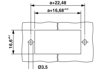
Для винтового крепления
