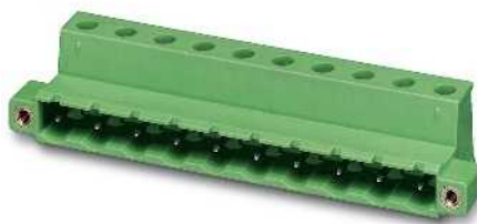
С резьбовым фланцем для крепления с помощью штекеров GMSTB
