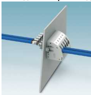
Серия PWO 16-POT: разъемы Push-in, до 76 А, без оранжевой кнопки PWO 16-POT... Стр. 604
