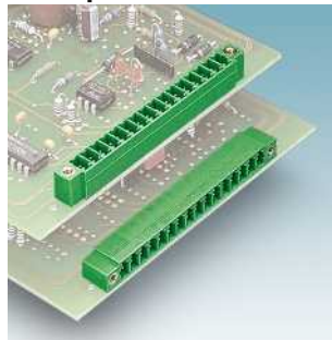
Ответные части для пайки волной припоя, шаг выводов 3,5 / 3,81 мм, подключение параллельно и перпендикулярно печатной плате MC(V) 1,5/...-G(F)-... Стр. 224
