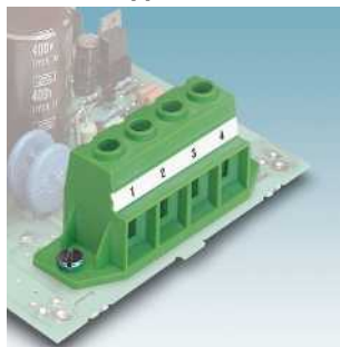
Серия MKDSP 25: винтовые зажимы, до 125 А, шаг 15 мм MKDSP 25... Стр. 455
